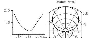
VSWR特性 ビームパターン
