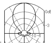
ビームパターン (垂直偏波 水平面)
