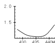
V SWR特性
